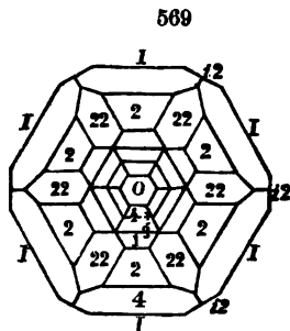
Vesuvius.
